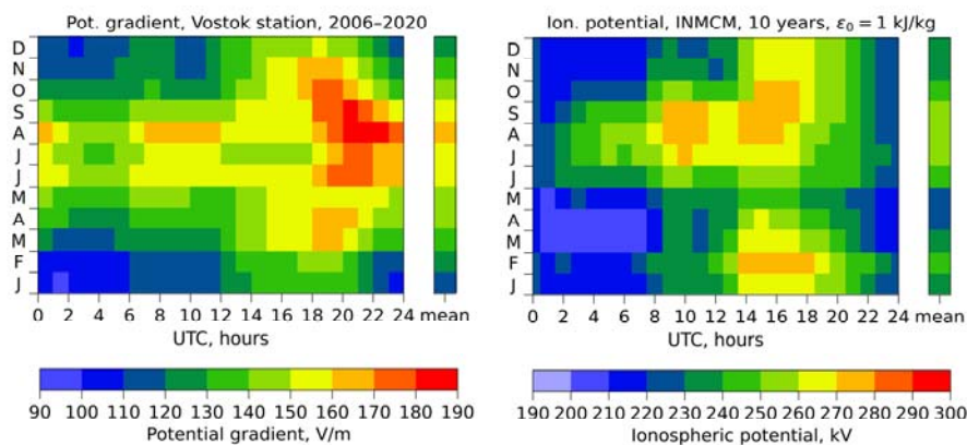
Рис. 1. Суточно-сезонная диаграмма параметров ГЭЦ постоянного тока по результатам измерений (левая панель) и по результатам моделирования (правая панель)
