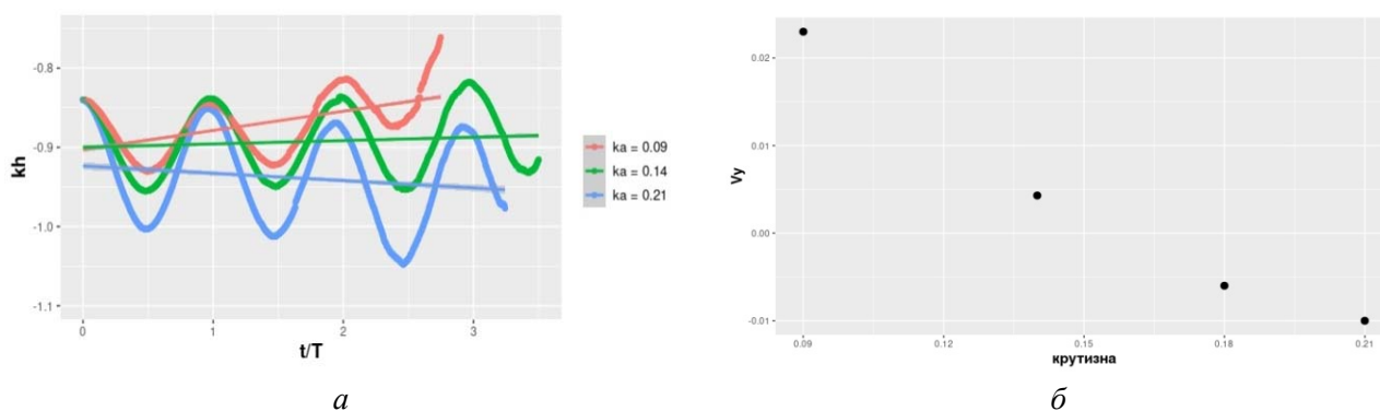
Рис. 2. Зависимость безразмерной вертикальной координаты пленки от безразмерного времени (в периодах волн) при различной крутизне волн ( а ) и зависимость скорости изменения вертикальной координаты пленки от крутизны волны ( б )
