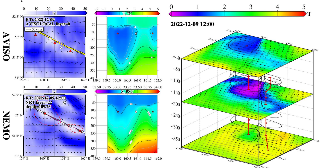
Рис. 1. Карта поля скорости течения на поверхности по данным AVISO и на горизонте 110 метров по данным реанализа GLORYS12V1 (левая колонка). Вертикальный профиль температуры и солёности на основе GLORYS12V1 (центральная колонка) и псевдотрехмерное изображение вихрей (справа), где черными линиями показаны контуры вихрей, полученные алгоритмом AMEDA. Красный треугольник обозначает центр антициклонического вихря на заданном горизонте. Красные линии – вихревые оси
